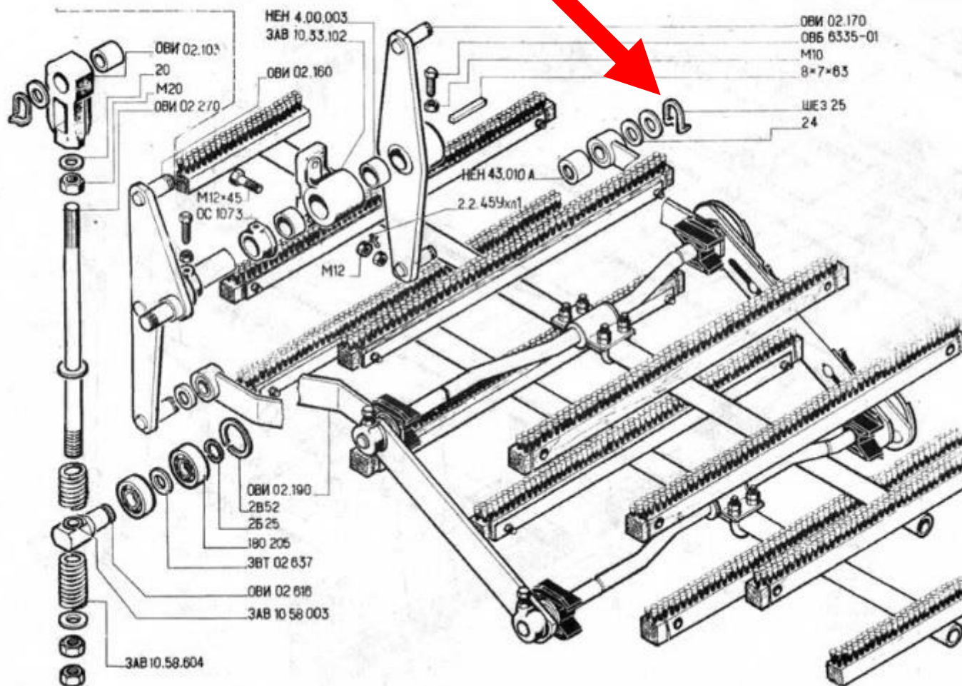
Рис. 12. Механизм очистки решет ОВИ 02.150.
